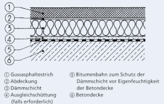
Schwimmender Gussasphaltestrich auf Massivdecke
